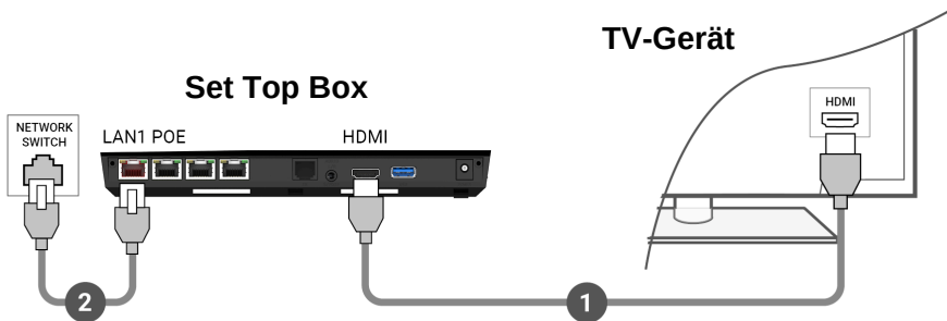
Abbildung 2: Kabelverbindungen - PoE
